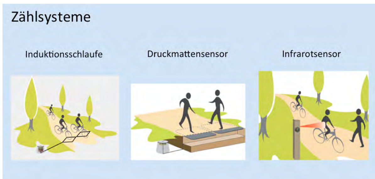
Abbildung 3.1.: Zählsysteme, Bilder übernommen von Eco-Compteur (2013)
