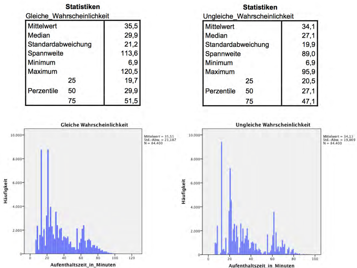
Abbildung 7.1.: Deskriptive Statistiken und Histogramme für die Simulationsergebnisse der Methoden der gleichen Wahrscheinlichkeit (links) sowie der ungleichen Wahrscheinlichkeit (rechts)
