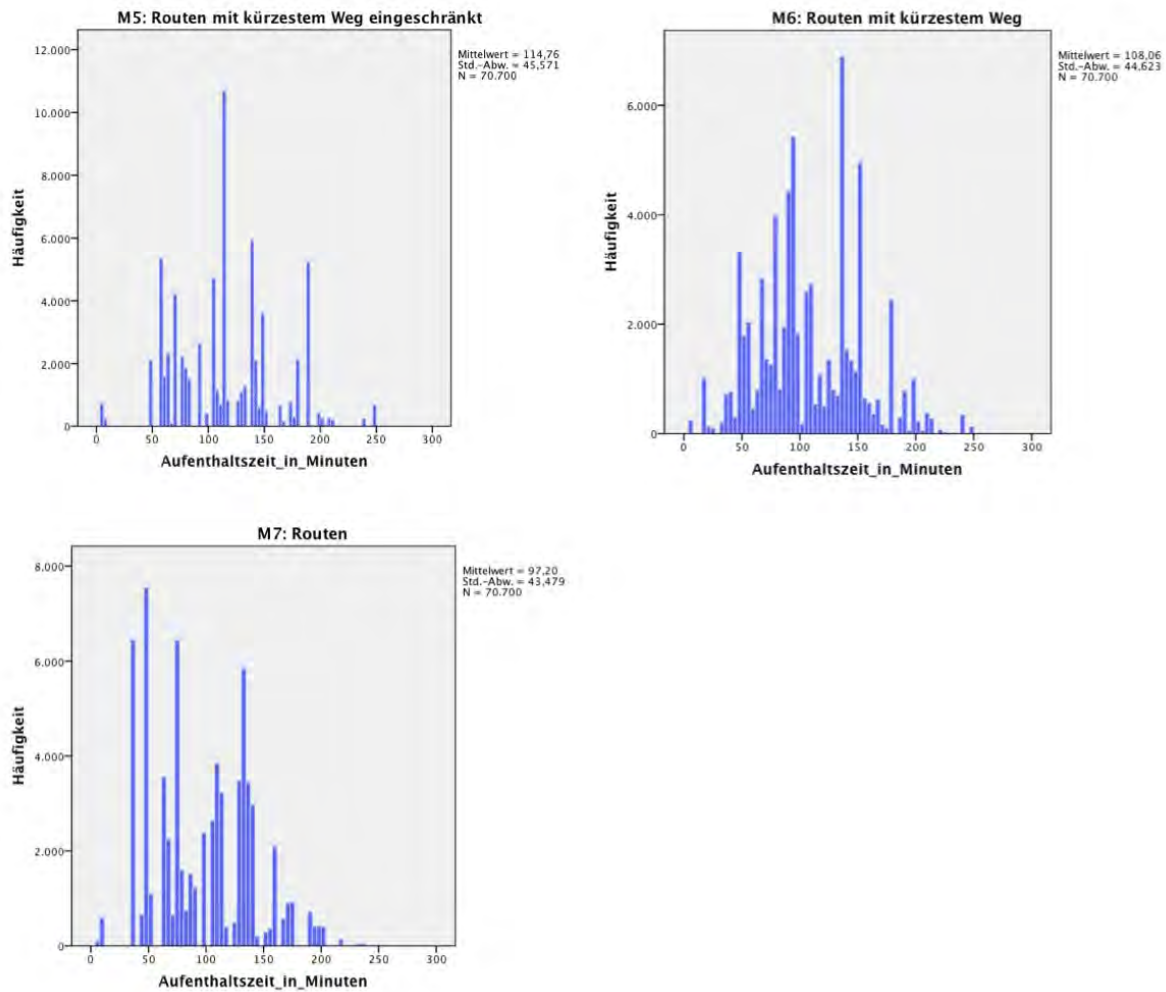
Abbildung 7.2.: Deskriptive Statistiken und Histogramme für die Simulationsergebnisse der verschiedenen Methoden für den Sihlwald
